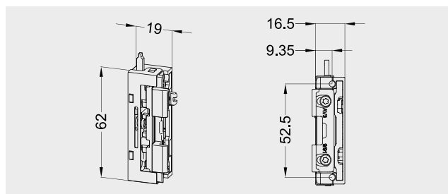
Dimensions principales
