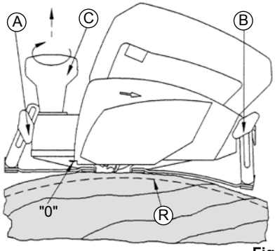
Fig. 4 SUPERFICIE CONVEXA
