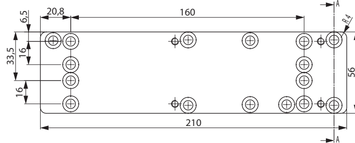
Plaque de montage plate de rechange A124
