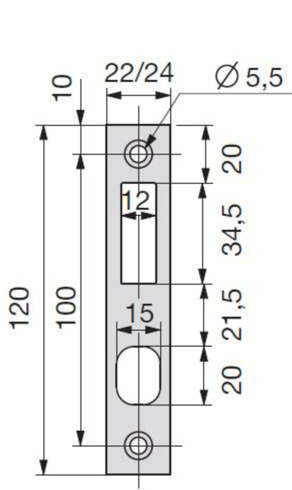
Gâche H et B. ép: 2,5 mm
