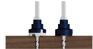
TerrassenFix® Bohrsenker BS 5 & BS 6
