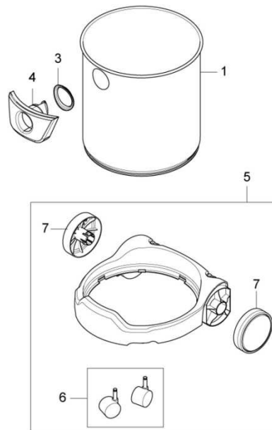
NOMENCLATURE VUE ECLATEE CUVE DCi35-S (VUE 02)
