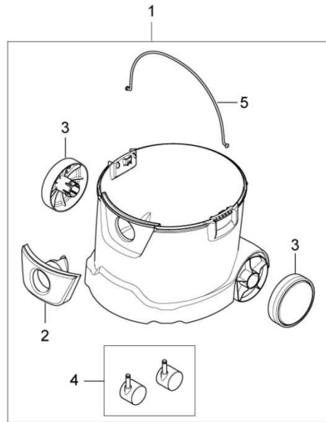
NOMENCLATURE VUE ECLATEE CUVE DCP25/DCP25-S (VUE 01)
