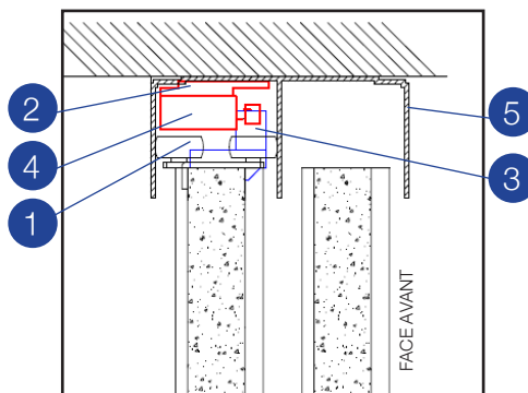
DÉTAIL SECTION VERTICALE
