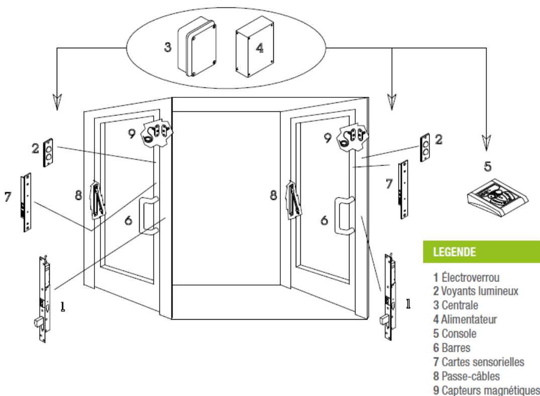
SYSTÈME D'INTERBLOCAGE AVEC ÉLECTROVERROUS SÉRIE MAXIMA
