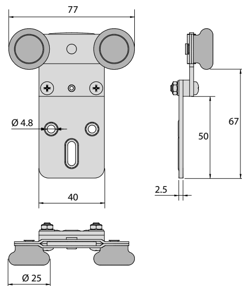
Monture 38 Hanger 38 Rollapparate 28 Roldana 28
