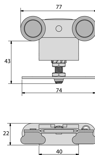
Monture 38 C Hanger 38 C Rollapparate 38 C Roldana 38 C
