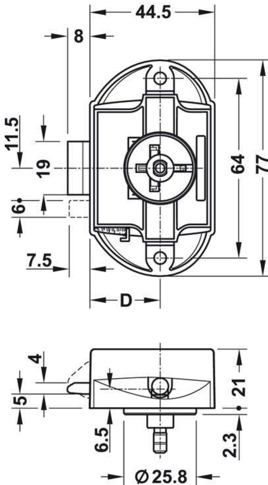
Schéma de la serrure bouton poussoir
