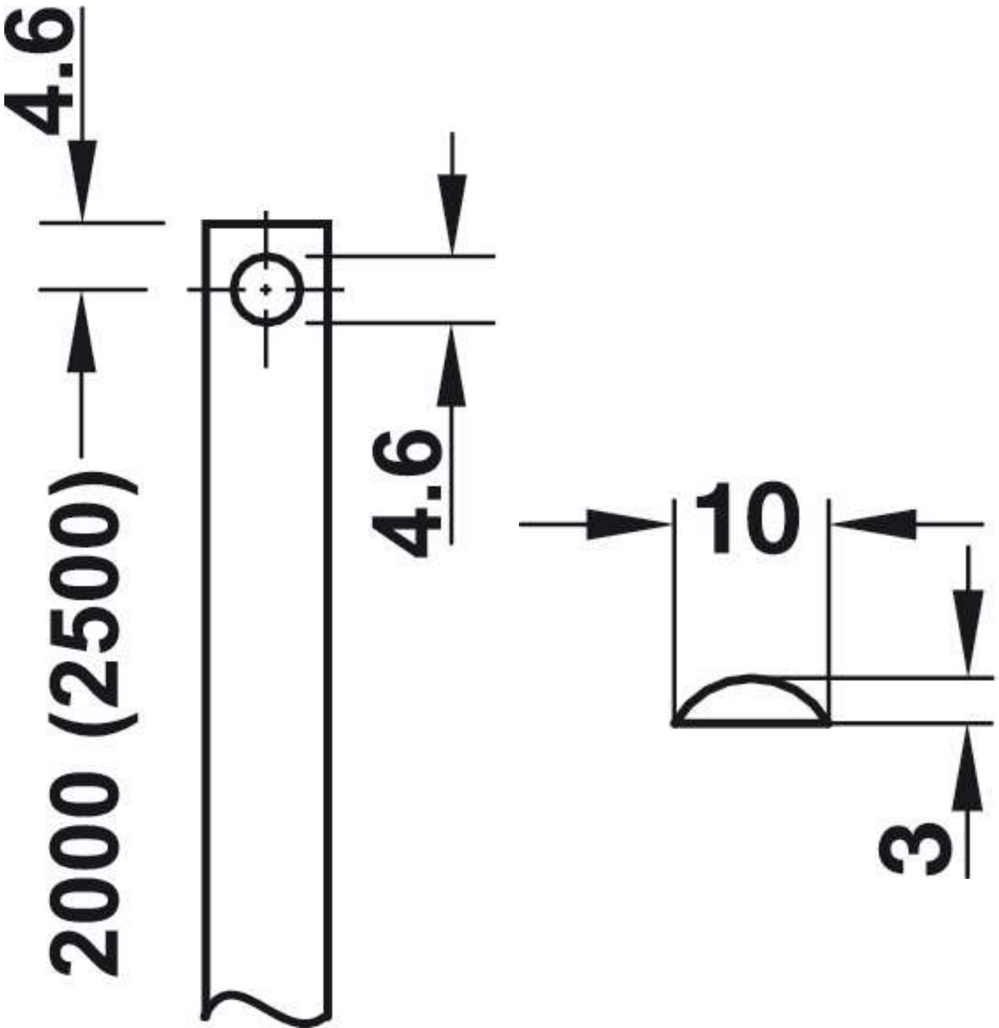
Schéma de la tringle plate
