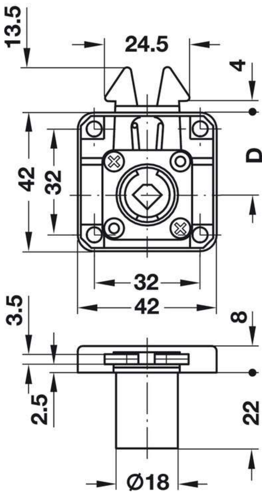
Schéma de la serrure à volet roulant – à appliquer
