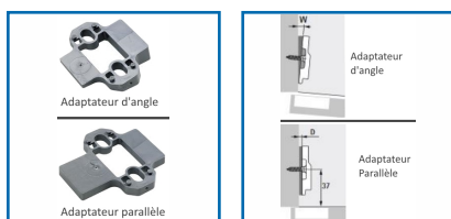
Adaptateur parallèle
