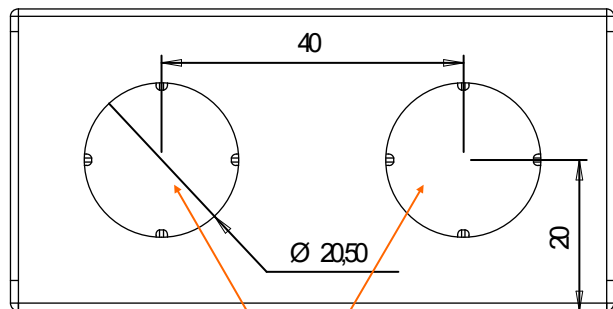
Opércules amovibles pour passage de câbles Pre-pierced openings for cable insertion Ausbrechbare Öffnungen für Kabeleinführung Afneembare openingdelen voor het overgang van kabels
