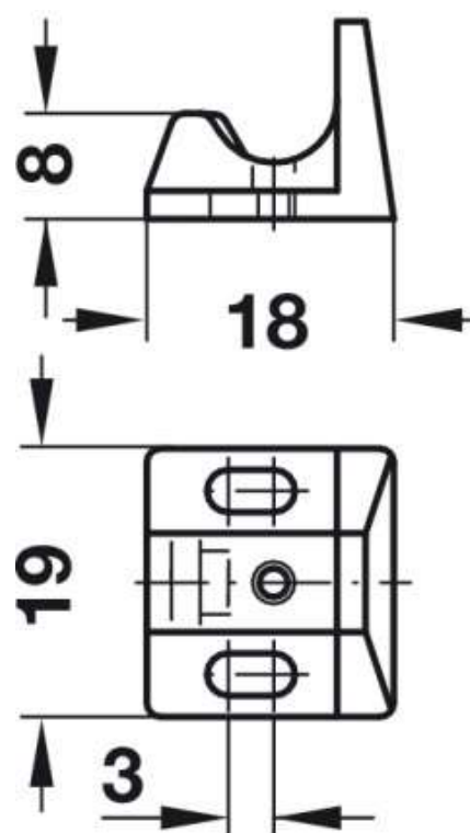
Schéma de la gâche pour le loqueteau Quick
